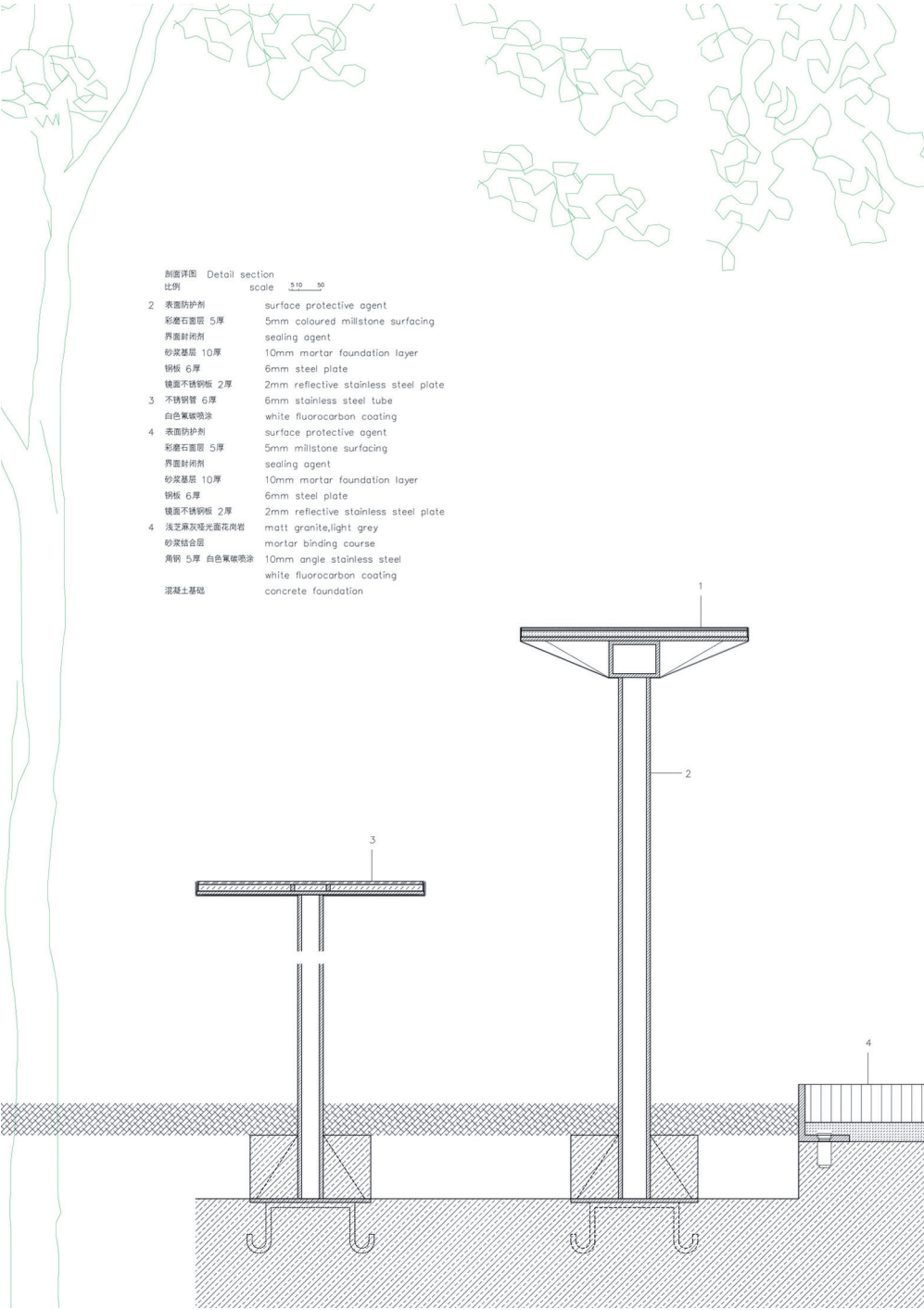
2 节点图 Section
